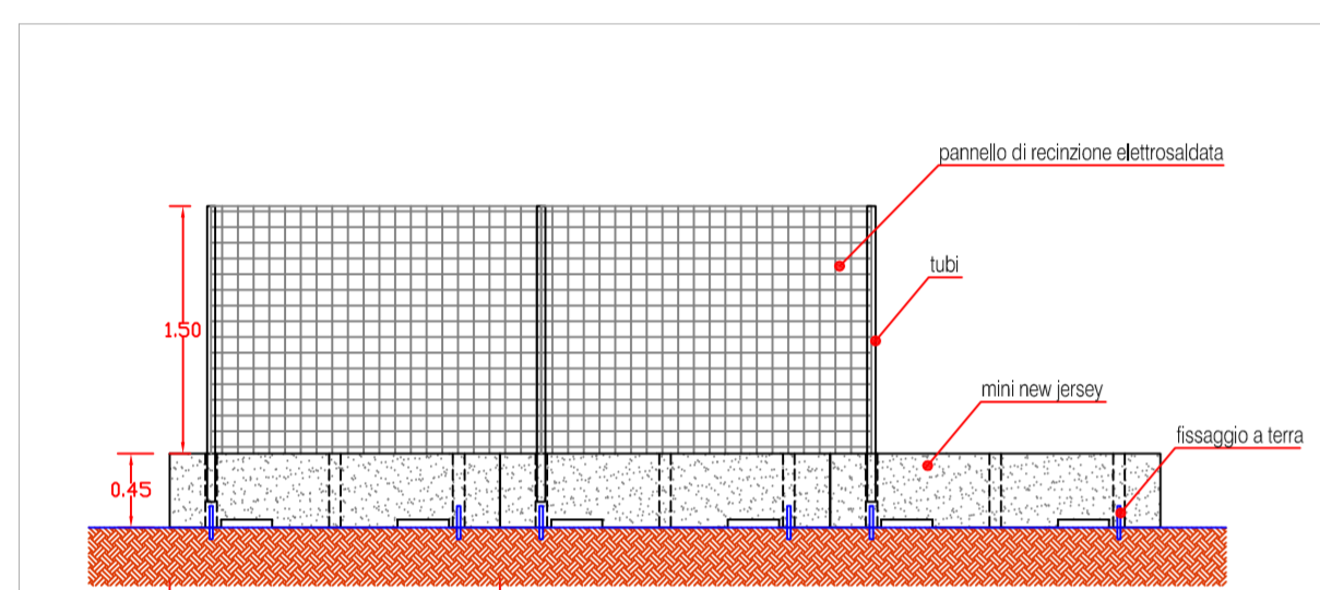
Particolare recinzione di cantiere scala 1:50
